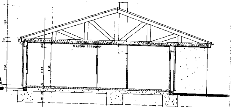
COUPE
